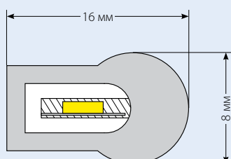
Поперечное сечение светодиодной ленты ULS-N21 NEON
