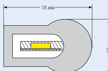
Поперечное сечение светодиодной ленты ULS-N22 NEON RGB
